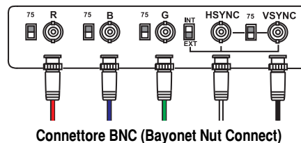
Connettore BNC (Bayonet Nut Connect)
